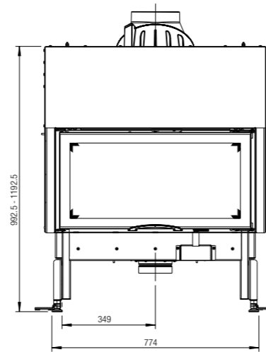
Maßstab 1:20
